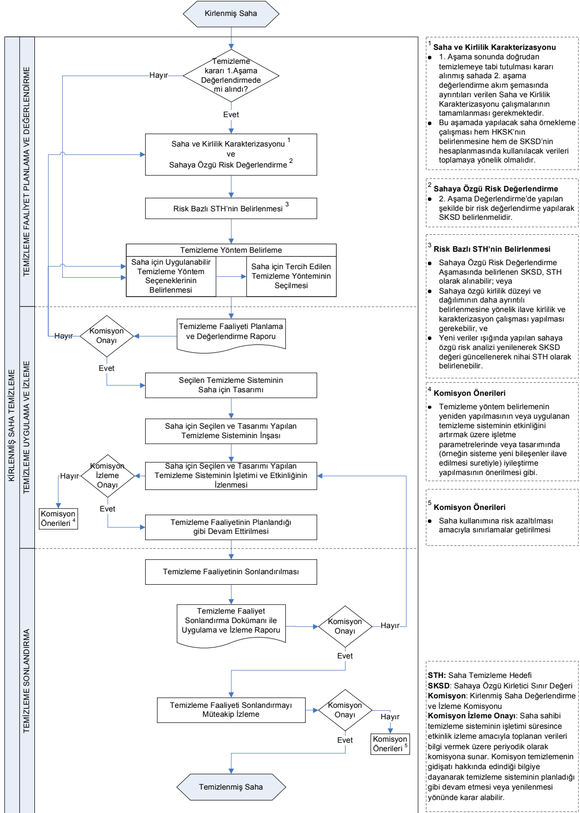
Şekil 1.1. Kirlenmiş Sahalar Temizleme Sistemi Ayrıntılı Akım Şeması
