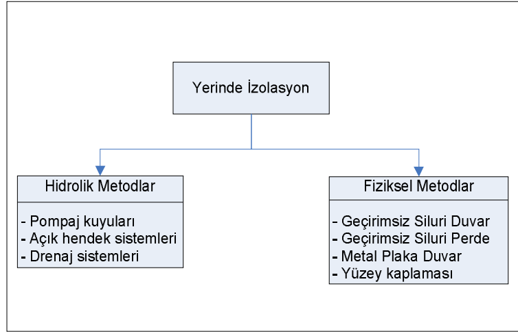
Şekil 2.5. Yerinde İzolasyon için Kullanılabilecek Genel Teknoloji Seçenekleri
