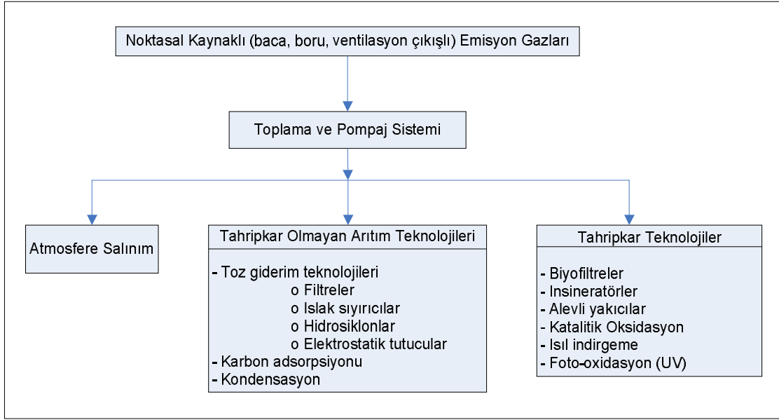
Şekil 2.4. Emisyon Gazları için Kullanılabilecek Genel Arıtım Seçenekleri
