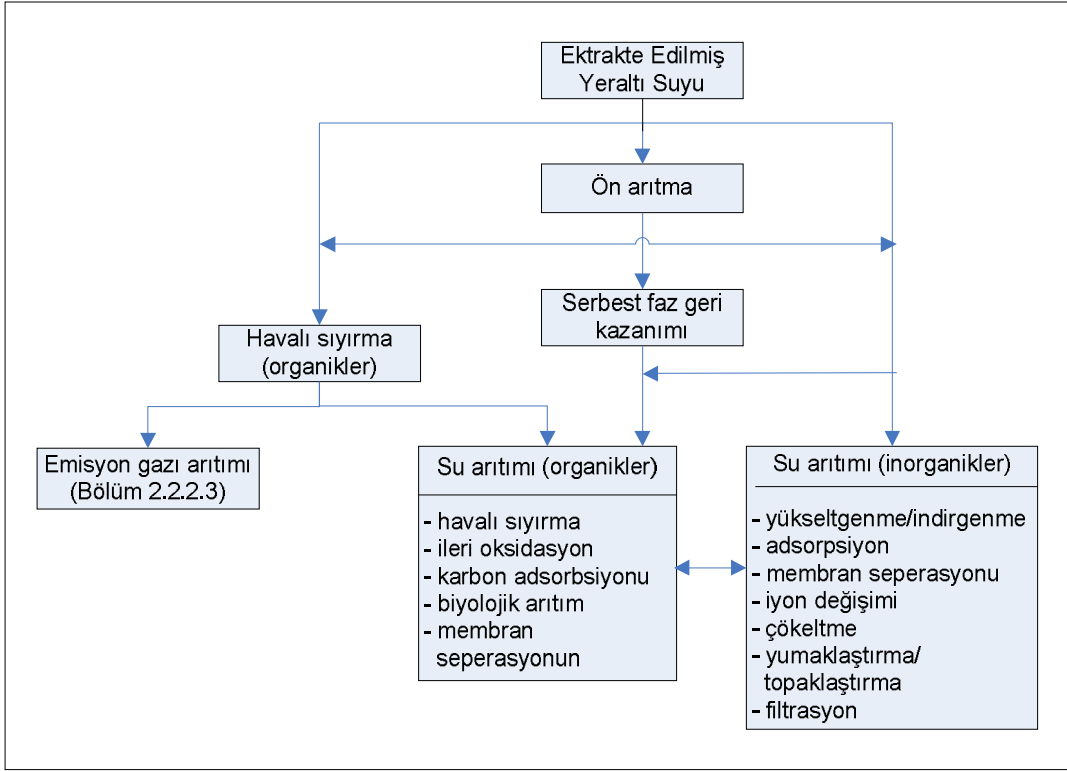
Şekil 2.3. Akiferden Ektrakte Edilmiş Yeraltı Suyunun Arıtım Ařamaları ve Her Ařamada Kullanılabilecek Genel Arıtım Çeřitleri
